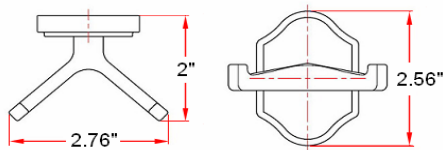
robe hook
