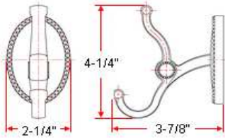
robe hook
