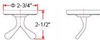
robe hook
